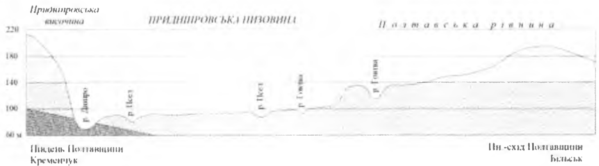
Рисунок 1.2 – Схематичний профіль через поверхню Полтавської області
